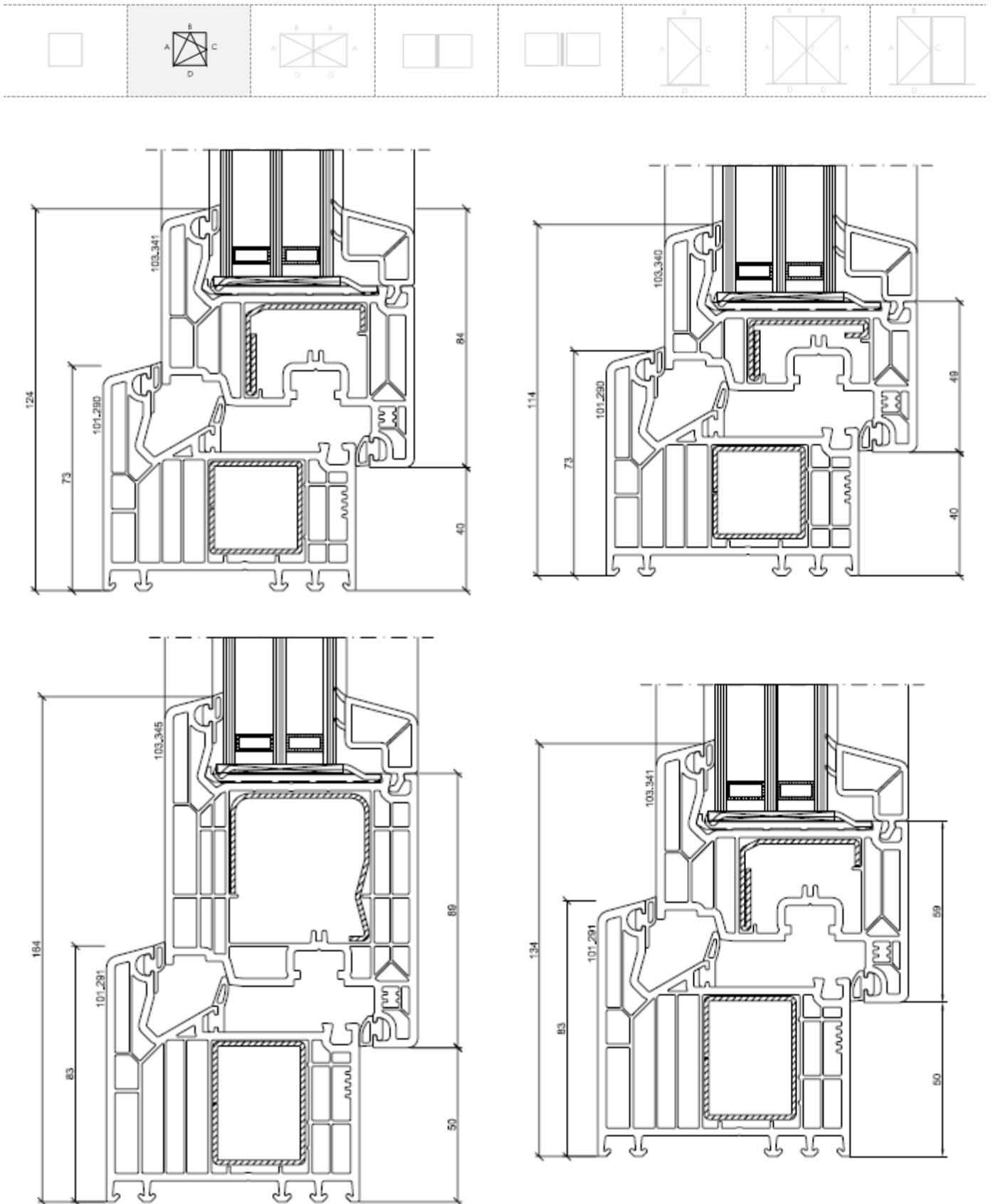
Figuur 7b: Typesnede draai-kip venster
