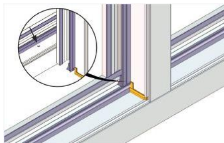
Mechanische T-verbinding zonder zijstukken
