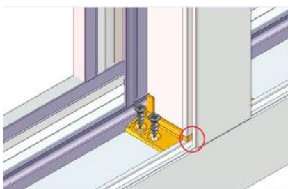
Mechanische T-verbinding met zijstukken
