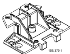
Mechanische T-verbinding met zijstukken
