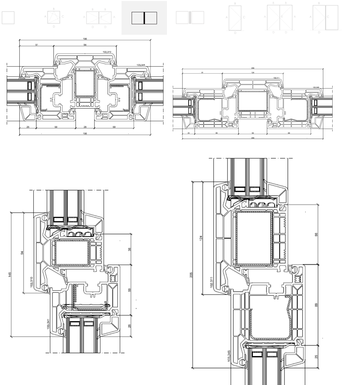
Figuur 7d: Typesnede samengesteld venster
